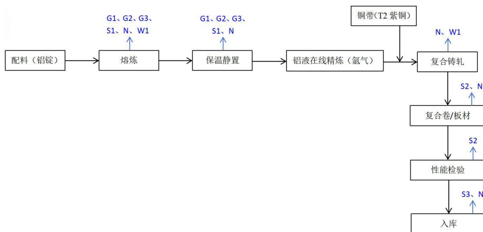
图 2-3 铜铝复合材料生产工艺流程及产污环节图
