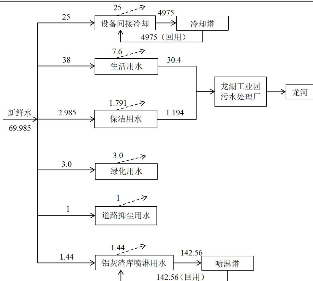
图 2-1 项目水量平衡图（单位：t/d）
