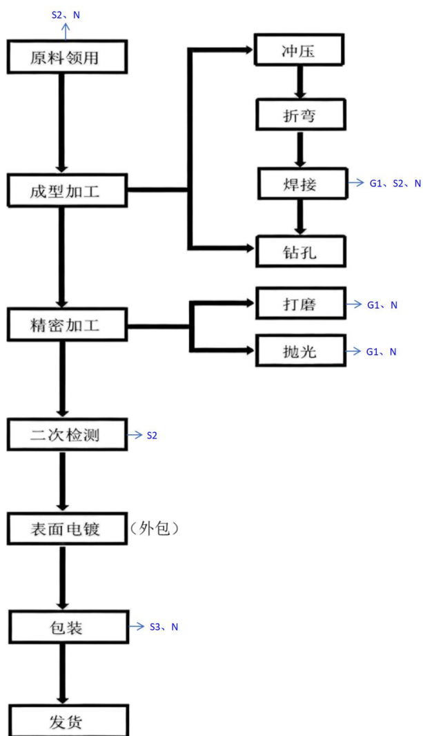
图 2-4 材料深加工工艺流程及产污环节图
