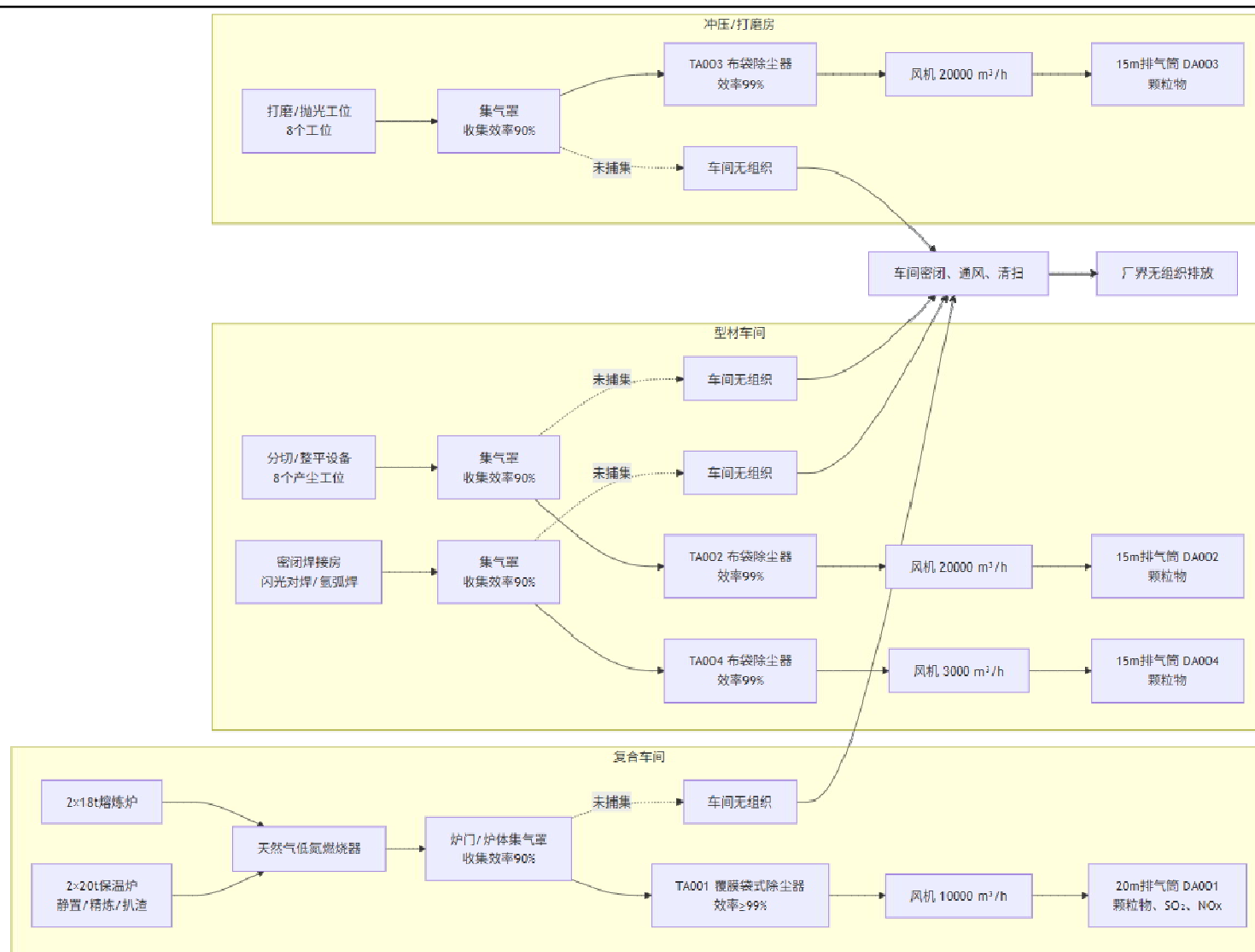
图 4-1 本项目废气走向示意图
